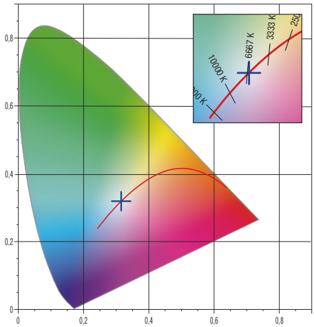
FARBWIEDERGABE – TM-30
